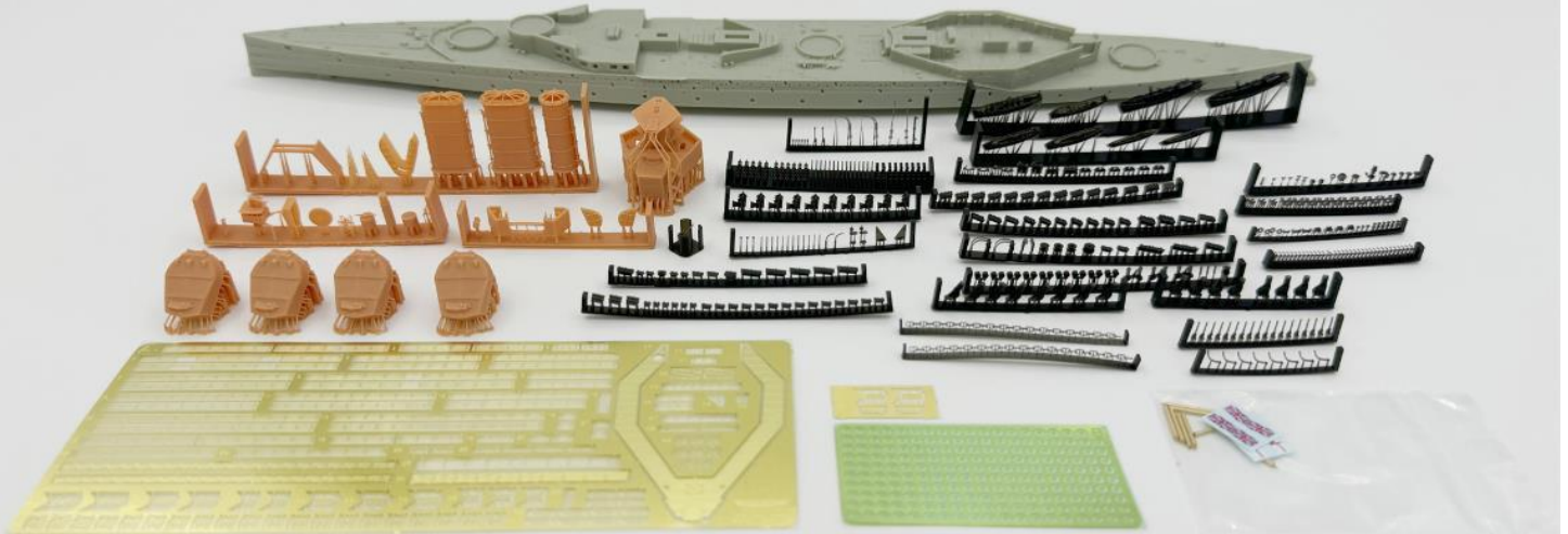
TRFM70011WLのパーツ構成
