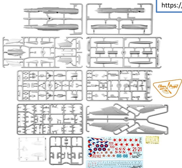
CPU72056 キットパーツ の構成です
