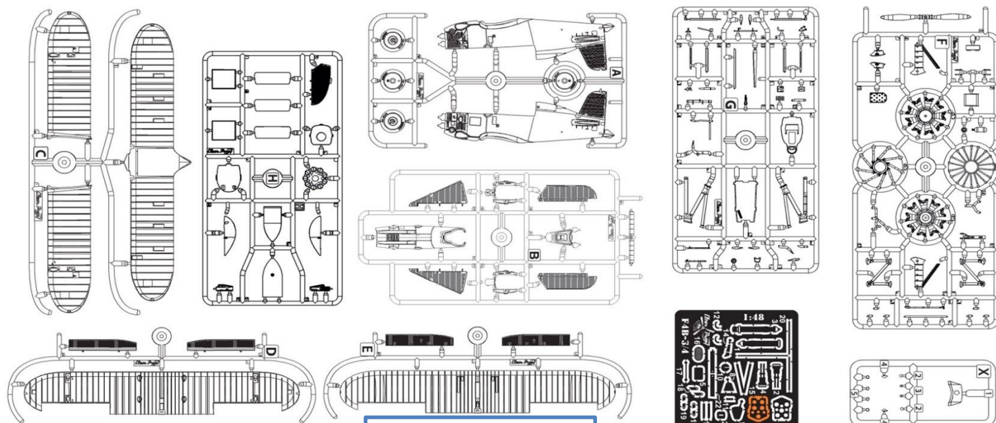
キットパーツの構成です
