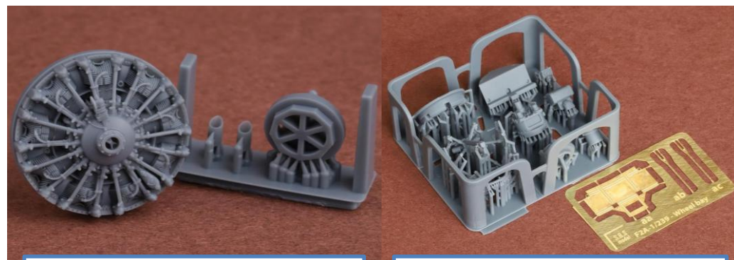
エンジン・排気管パーツの構成です
