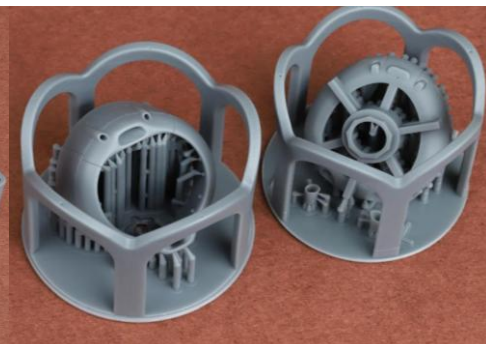
カウリングパーツの構成です
