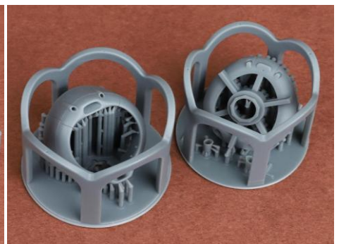
カウリングパーツの構成です
